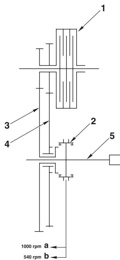
VERSION 2 DREHZAHLEWERTE
