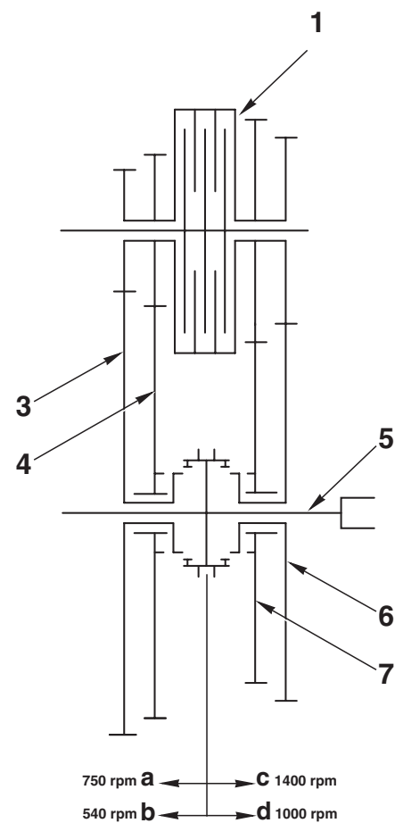
VERSION 4 DREHZAHLEWERTE
